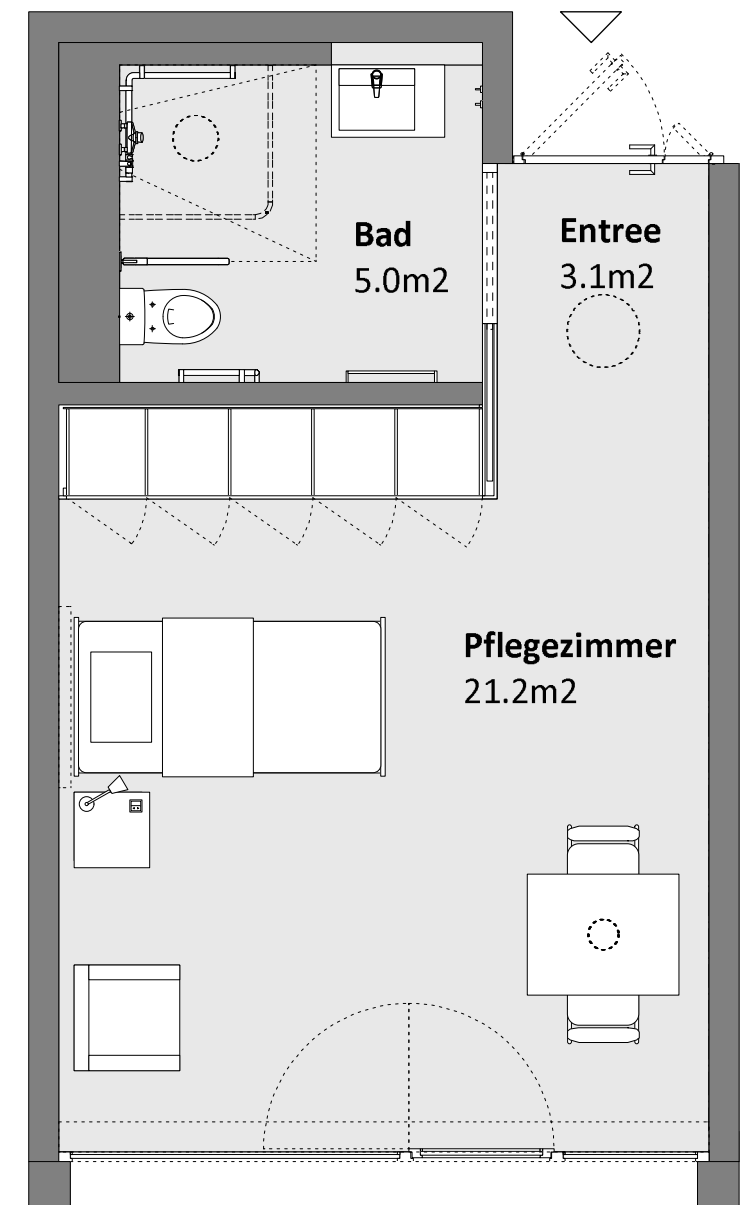
Grundriss Pflegezimmer
